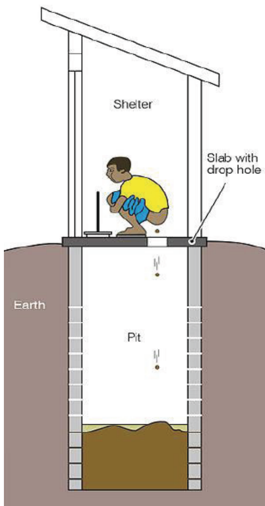
Een pit-latrine
